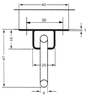
Einbaumaße Installation dimensions Cotes de montage
