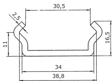
Außenprofil 1207
